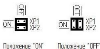
Рисунок 3 - Положение переключек на разъемах XP1 и XP2
